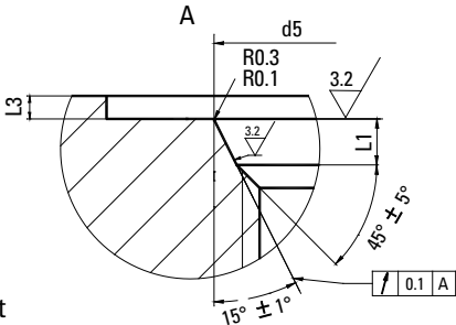
JIS B 2351 Port
