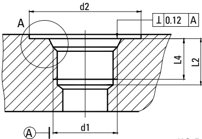
JIS B 2351 Port
